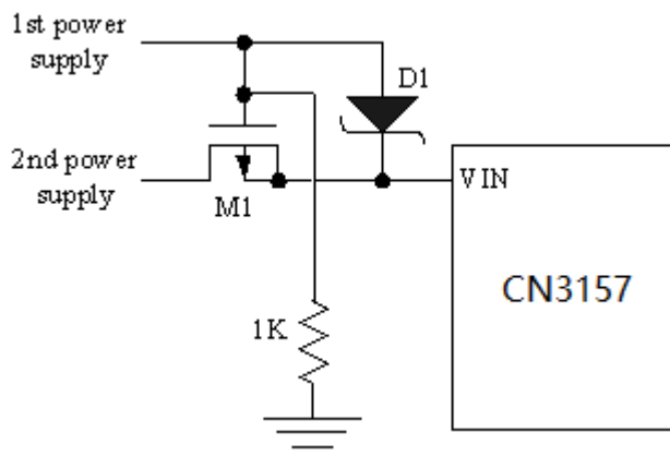
图6 同时使用两种输入电源供电
