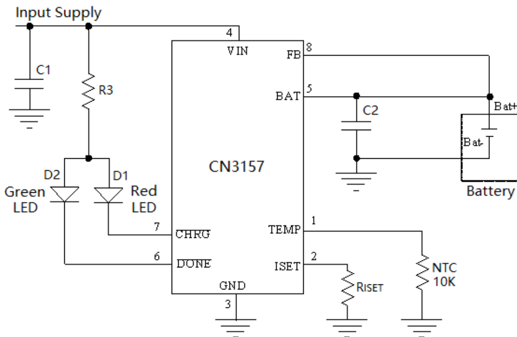
图 1 典型应用电路（恒压充电电压 3.63V）
